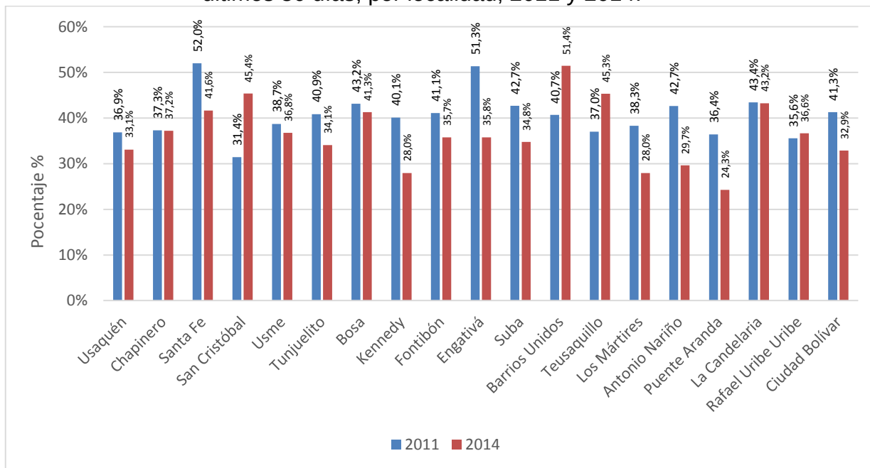
Gráfica 116. Bogotá. Niños y niñas menores de 5 años que tuvieron tos en los últimos 30 días, por localidad, 2011 y 2014.
