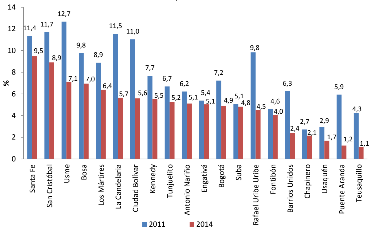
Gráfica 134. Bogotá. Porcentaje de hogares en los que algún miembro del hogar no consumió ninguna de las tres comidas uno o más días a la semana, según localidades, 2011 – 2014.
