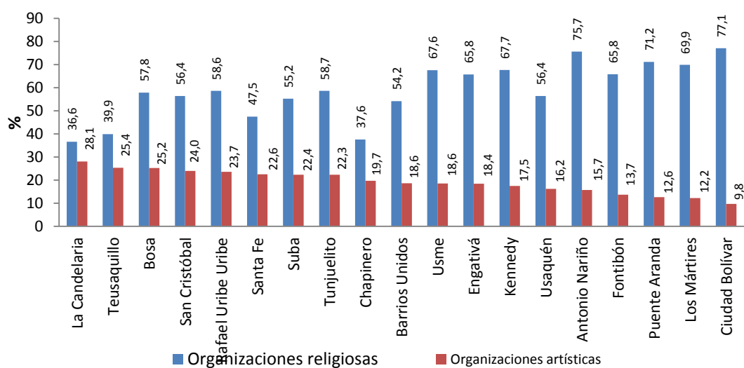
Gráfica 167. Bogotá. Participación de personas de 10 años y más en organizaciones religiosas y artísticas, según localidad, 2014.
