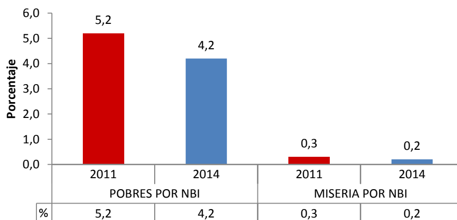
Gráfica 143. Bogotá. Porcentaje de pobreza y miseria por NBI, 2011 – 2014.
